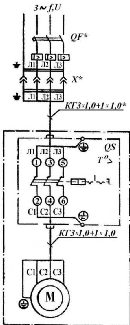
Рис. 10 Схема электрическая принципиальная установки компрессорной K25M1; K25M3
